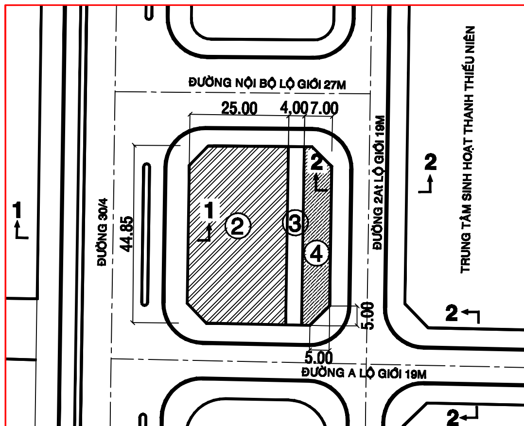
MẶT BẰNG ĐIỀU CHỈNH QUY HOẠCH TL 1/1000 PHÊ DUYỆT CỦA UBND THỊ XÃ TÂY NINH
