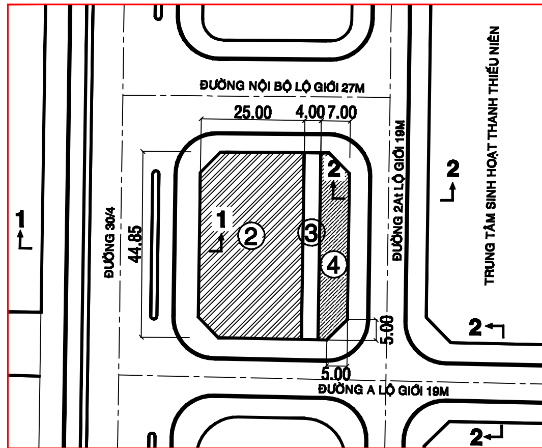
MẶT BẰNG ĐIỀU CHỈNH QUY HOẠCH TL 1/1000 THEO ĐỀ NGHỊ CỦA PHÒNG QUẢN LÝ ĐÔ THỊ
